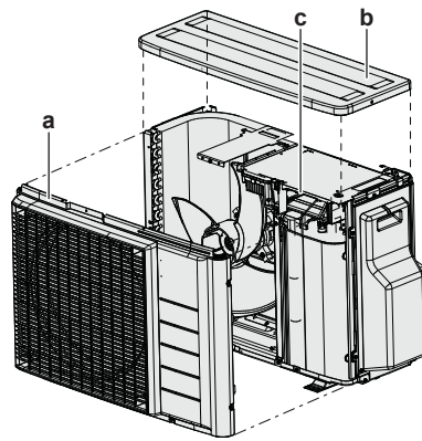
a Πρόσοψη b Επάνω πλάκα c Ακροδέκτης S99
